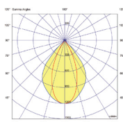
40x80° Optic
