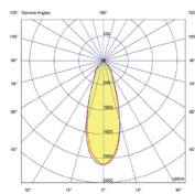
35° Optic
