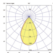
55° Optic
